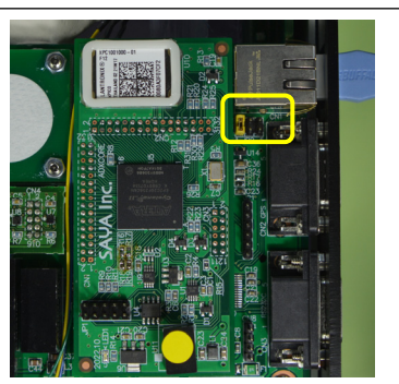
RS232C 921.6Kbps
